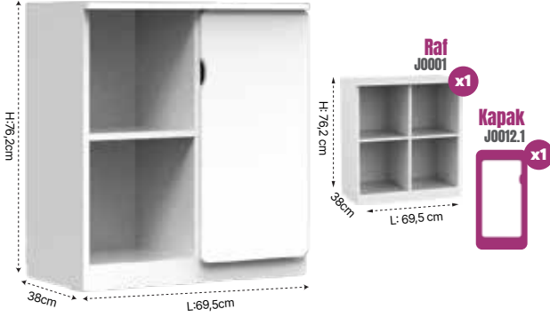
1 Kapaklı Raflı Dolap J0857
